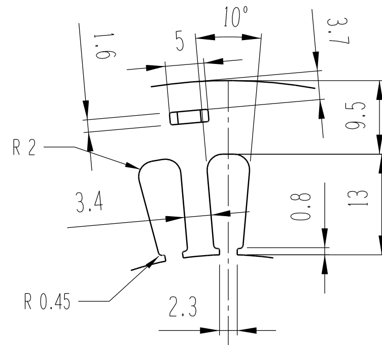
PART. B SCALA 2:1
